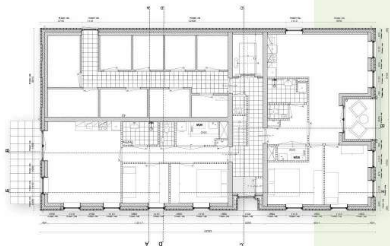
Begane grond 2 appartementen en 8 bergingen
