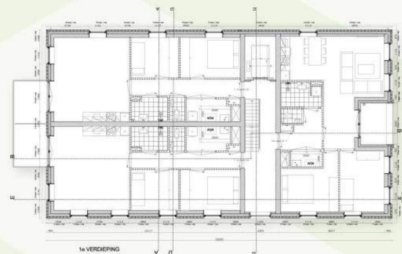
Eerste verdieping 3 appartementen
